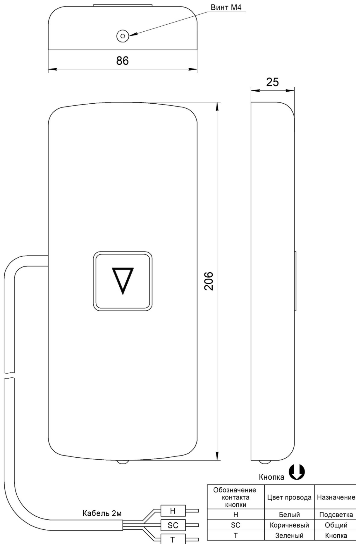
Рис.1 Внешний вид и габаритные размеры Вызывного поста ВП-1002-01
